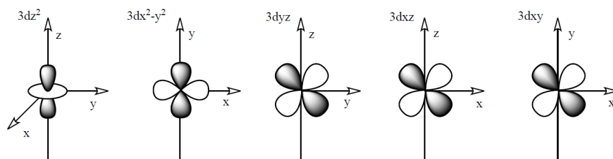
FIGURE 14.1 – Représentation conventionnelle des orbitales 3d
