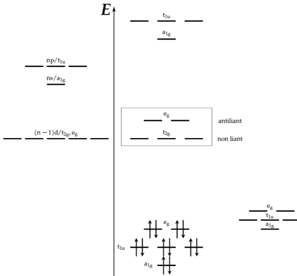
FIGURE 14.3 – Diagramme d'orbitales moléculaires de ML_6
