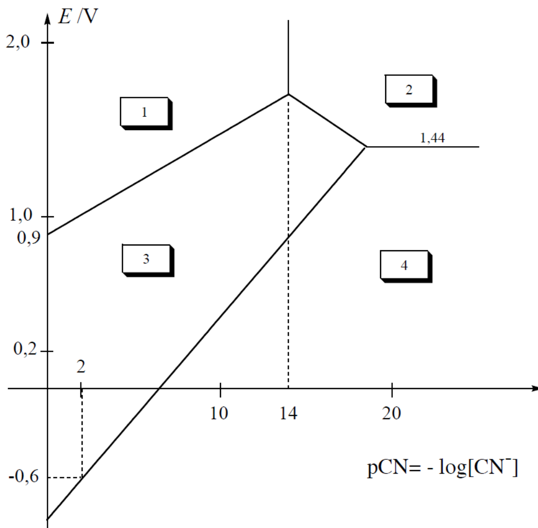
FIGURE 15.1 – Diagramme E-pCN de l'or
